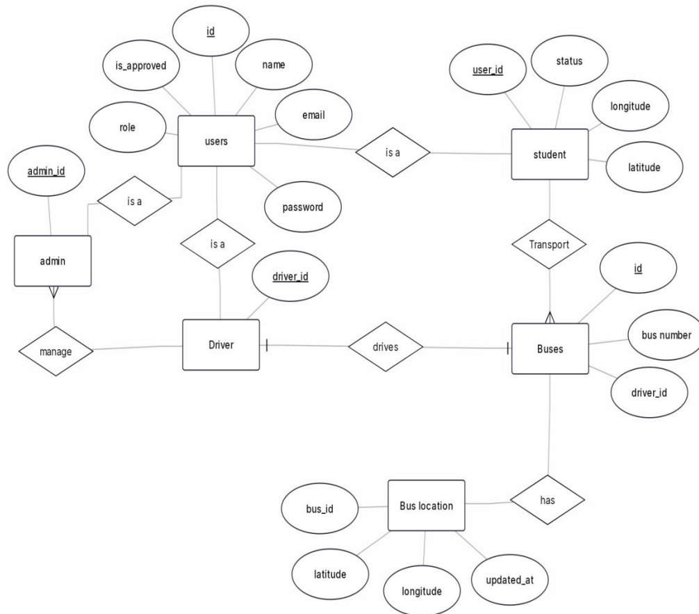
Figure 3.3: ER diagram
